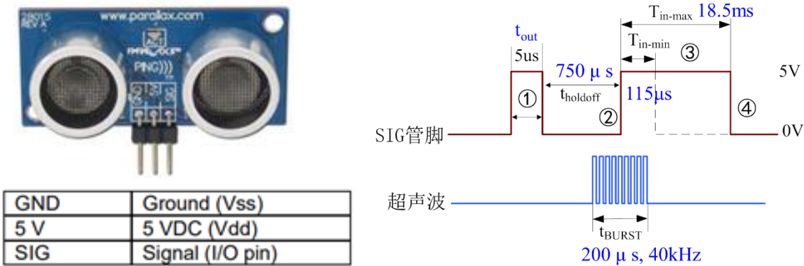
图 5 某超声波测距模块和其工作时序
